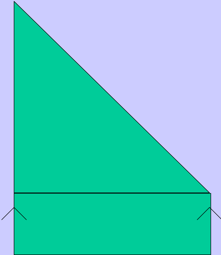
trapezium
